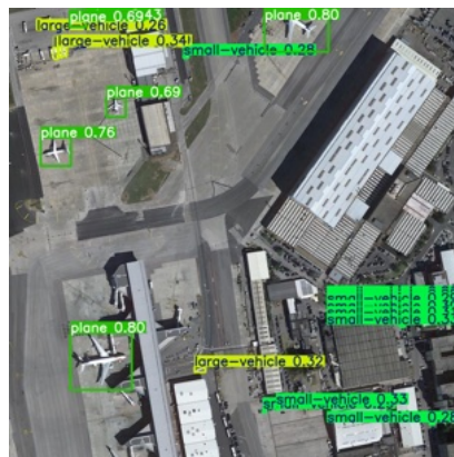
(d) Detections of the Model in Experiment 1
